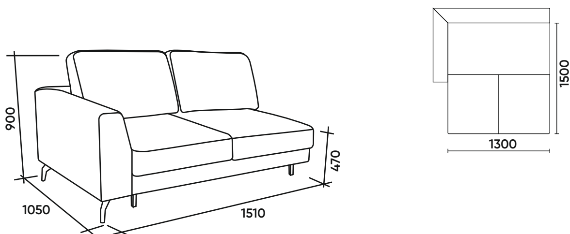
Диван боковой узкий левый УД2Л
