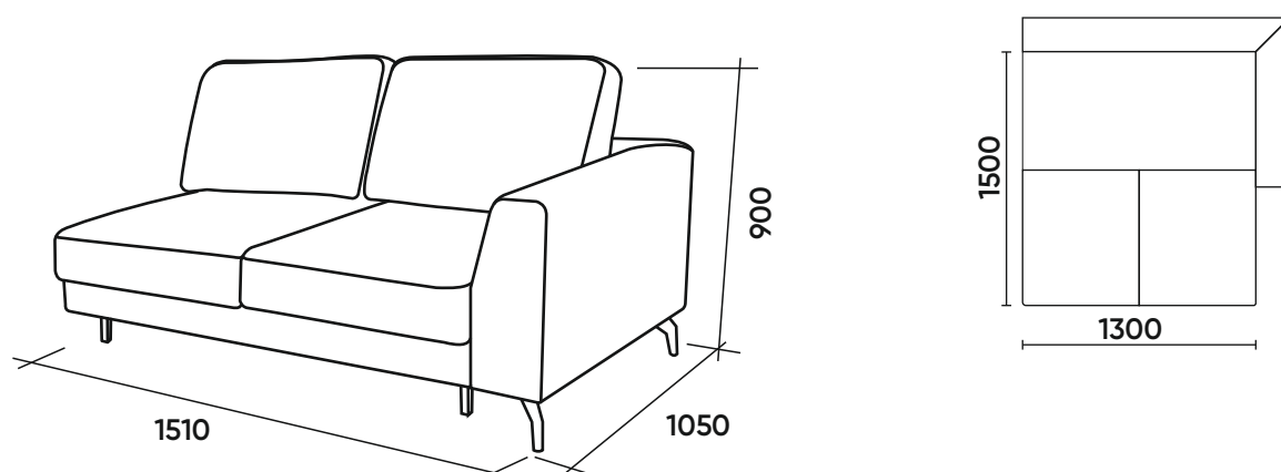
Диван боковой узкий правый УД2П
